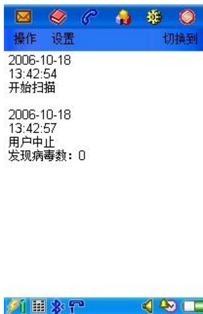
图 20 日志界面
