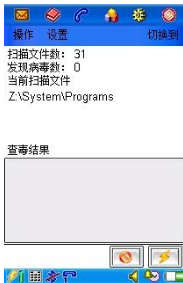
图 2 开始扫描
