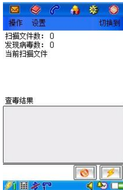
图 1 查杀病毒
